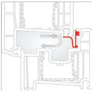
Kod naglog udara vjetra REHAU AirComfort zatvara se automatski prema Bernoullijevu principu
